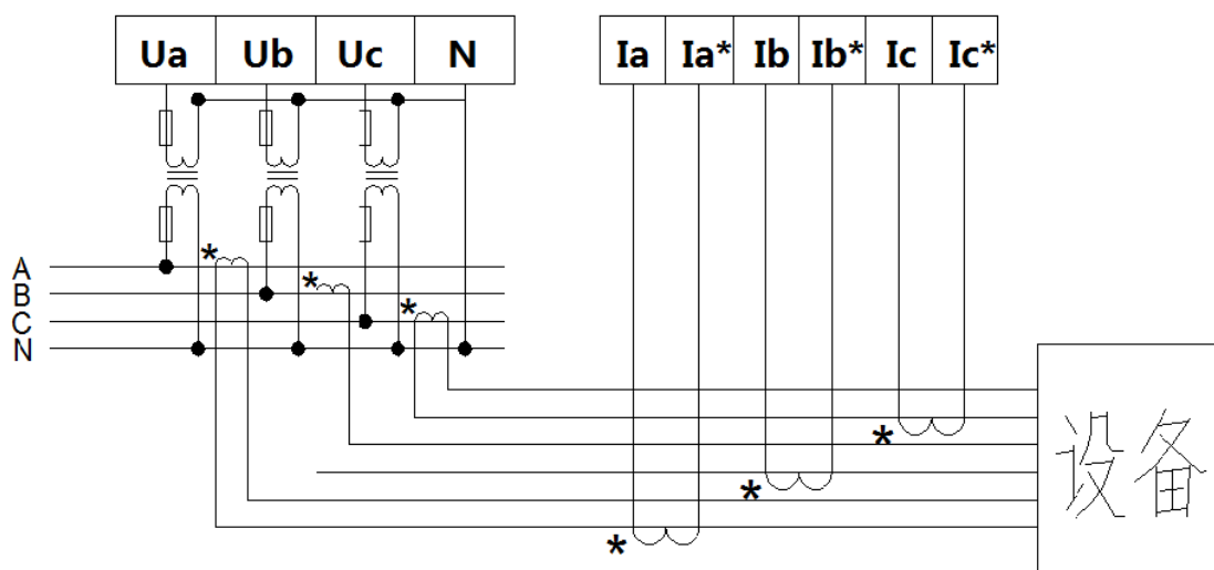
三相四线(电压、电流经互感器接入)
