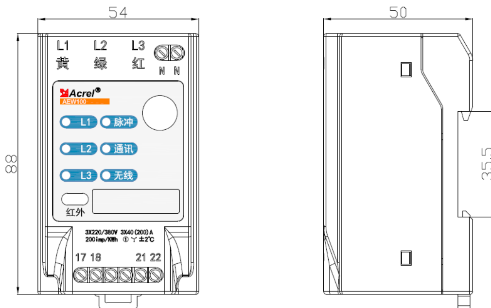
图 1 AEW100 尺寸图
